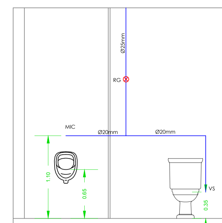
VISTA - BWC MASC. Escala 1:25
