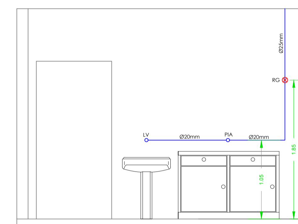
VISTA - COZINHA Escala 1:25
