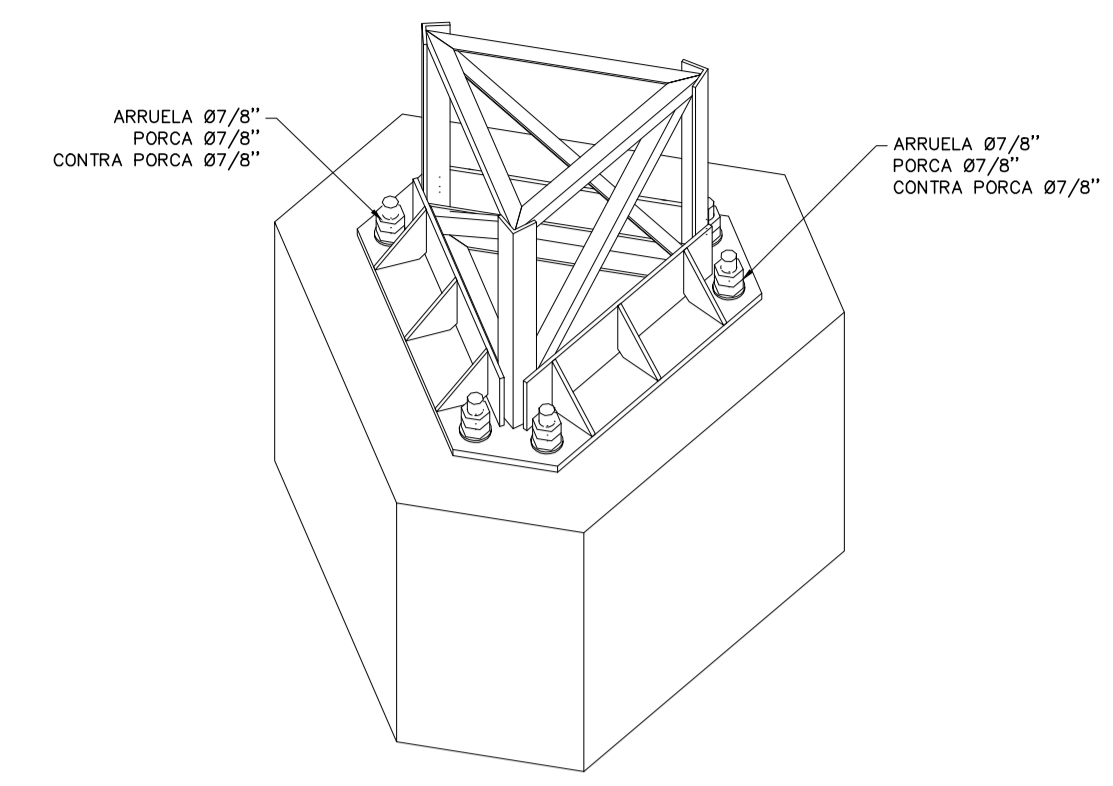
DETALHE DE FIXAÇÃO NA BASE DA TORRE ESC: 1/10
