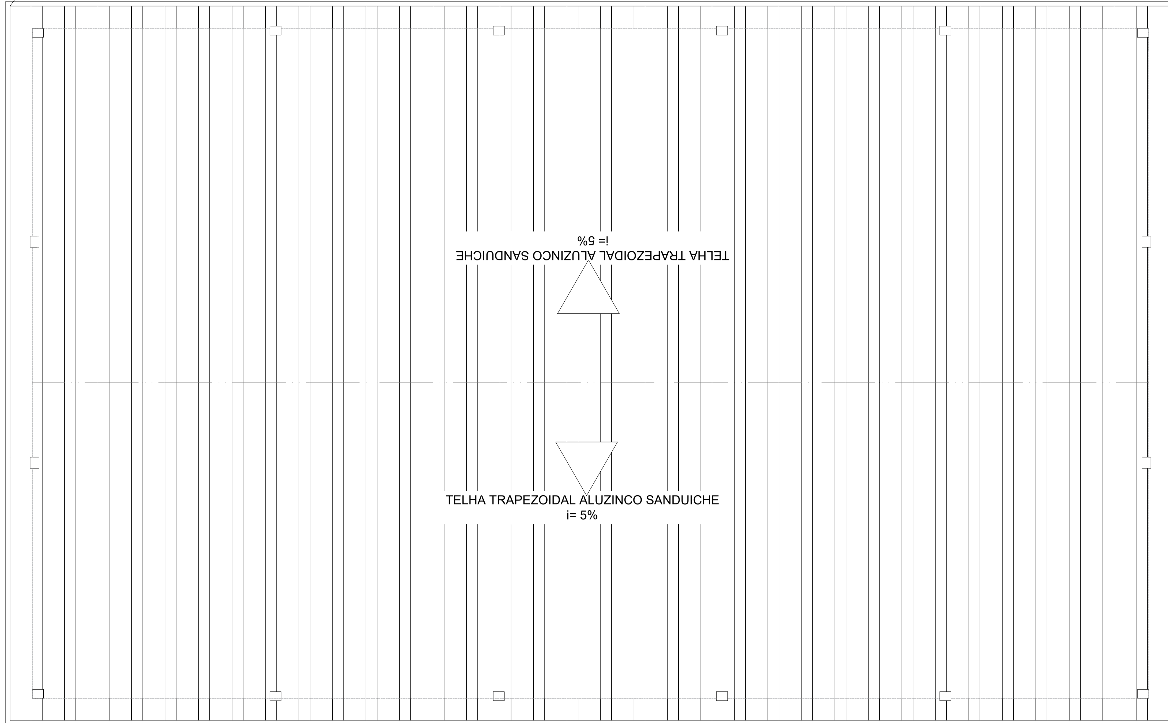
PLANTA DE COBERTURA ÁREA: 375,00m 2 ESCALA: 1/50
