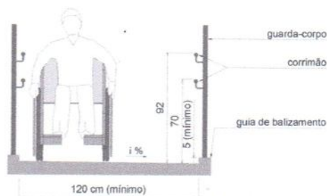
DETALHE CONSTRUTIVO DA RAMPA-VISTA FRONTAL
