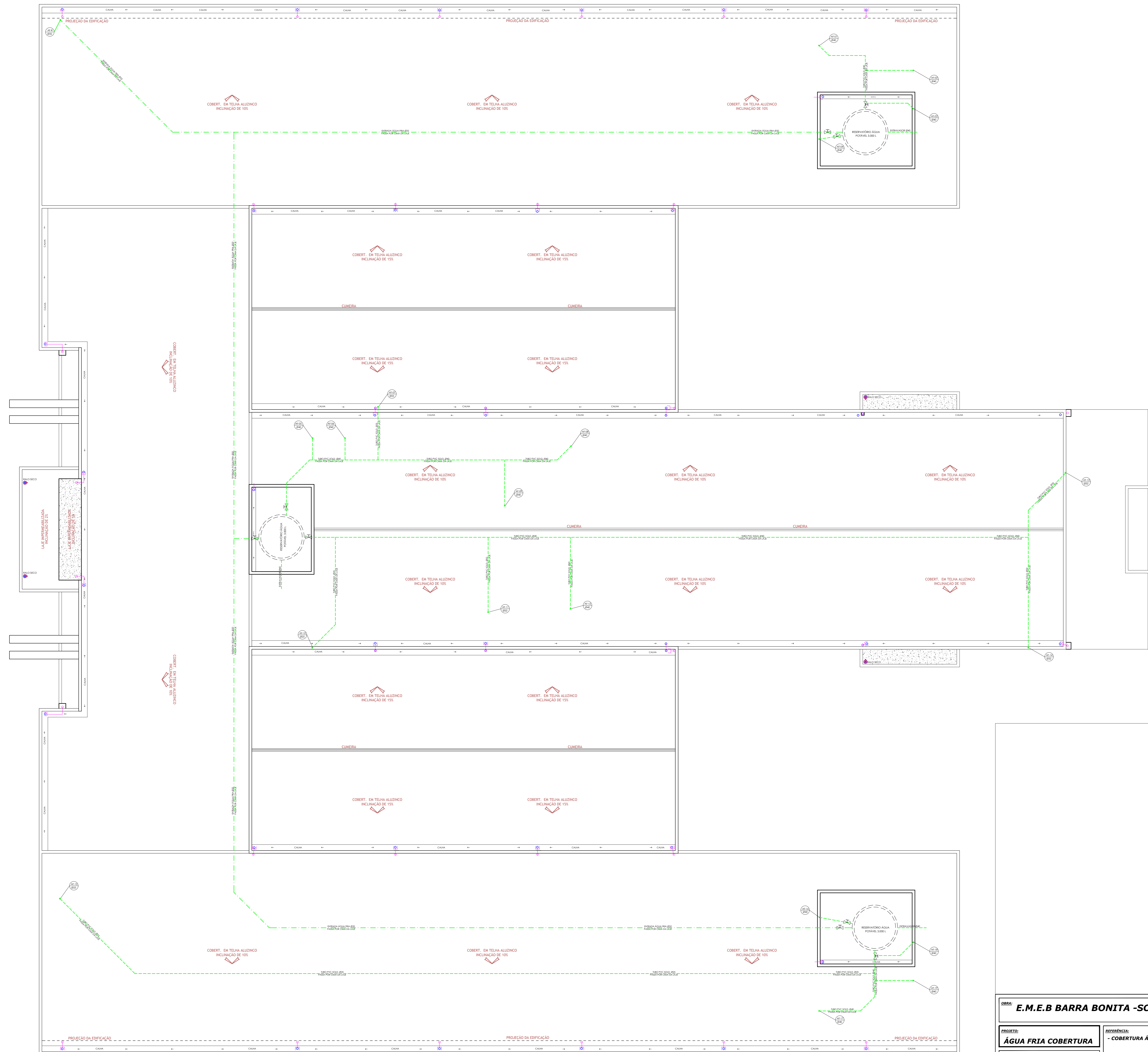
PLANTA DE COBERTURA PLUVIAL ESCALA: 1/75
