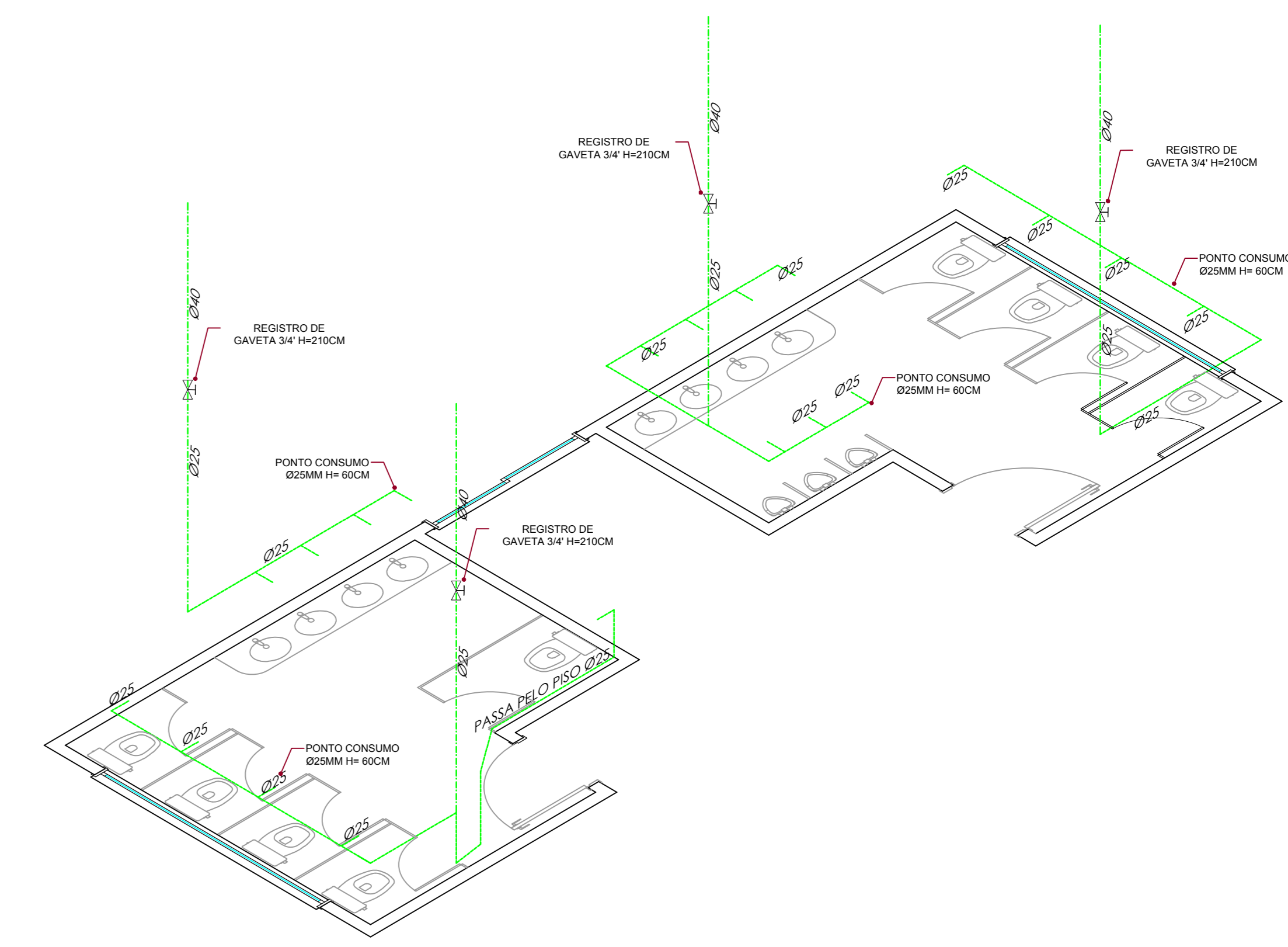
DETALHE ISOMÉTRICO PONTOS SANITÁRIOS ESCALA: 1/75
