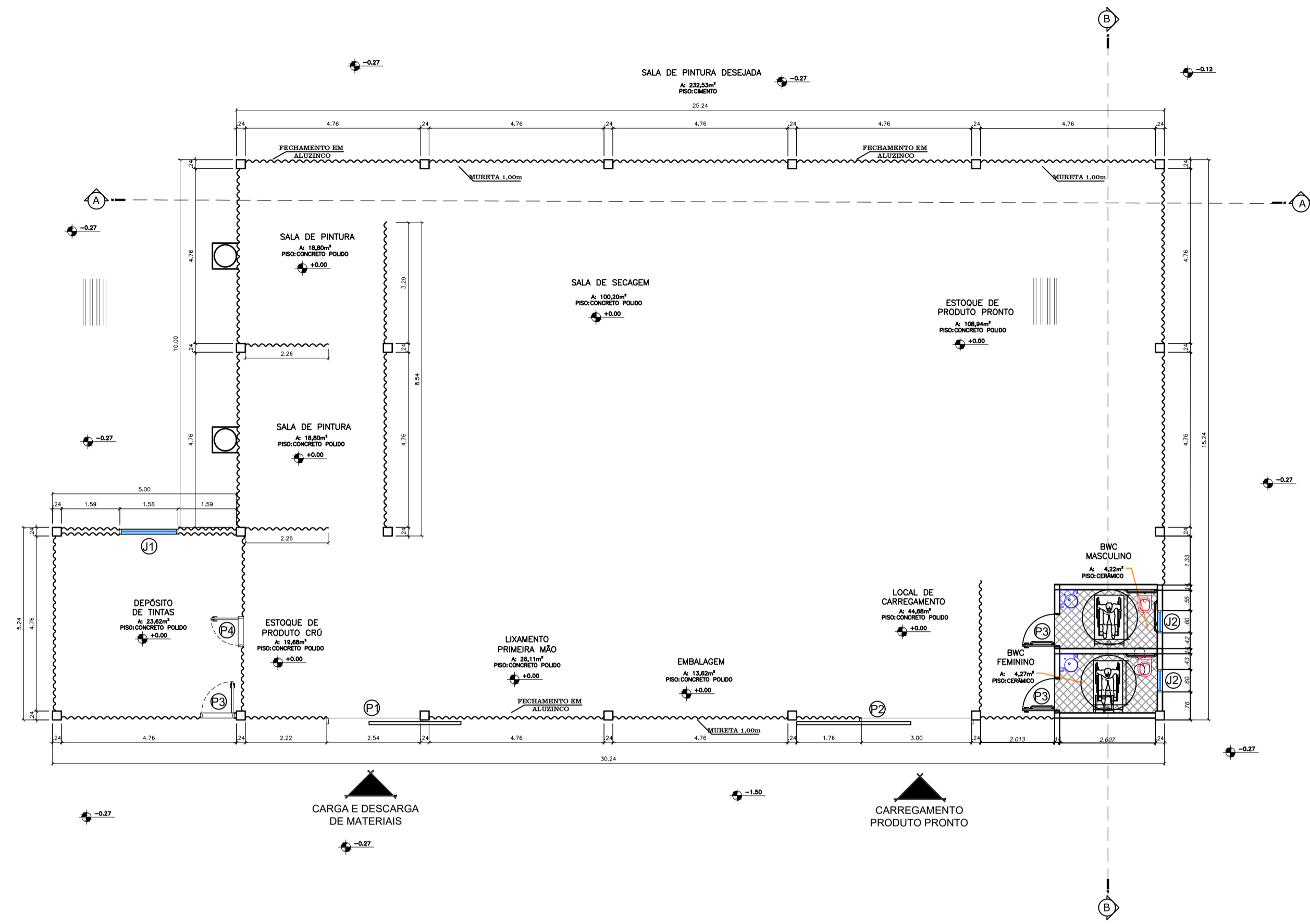
1 PLANTA BAIXA TÉCNICA ESCALA 1:50
